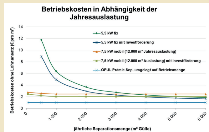
Abb. 2: Kosten der Separierung abhängig von der Jahresleistung bei durchschnittlicher Separatorleistung — Feststoff für Einstreu weniger geeignet. ÖPUL-Prämie von 1,5 Euro/m 3 auf Gesamtgülleanfall bei Verdünnung von 1:0,5 umgelegt.
