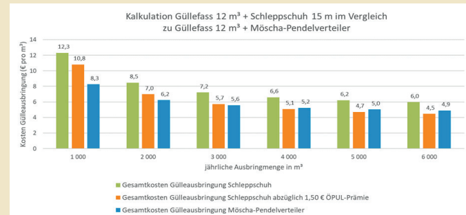
Abb. 2: Im direkten Vergleich der Ausbringsysteme „Schleppschuh“ und „Möscha-Pendelverteiler“ ist ersichtlich, dass sich bei Berücksichtigung der ÖPUL-Prämie „Bodennahe Gülleausbringung – Schleppschuh“ die Mehrkosten ab 3.000 m 3 ausgebrachter Menge pro Jahr gedeckt sind.
