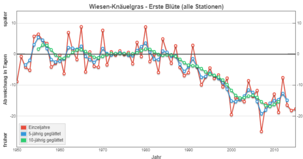
Diagramm 2: Zeitpunkt Knaulgras Ersten Blüte. Aus: PhenoWatch, ZAMG.
