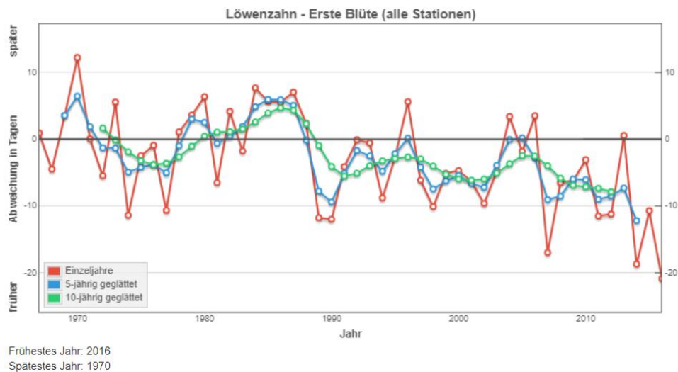
Diagramm 1: Zeitpunkt Erste Blüte Löwenzahn. Aus: PhenoWatch, ZAMG.
